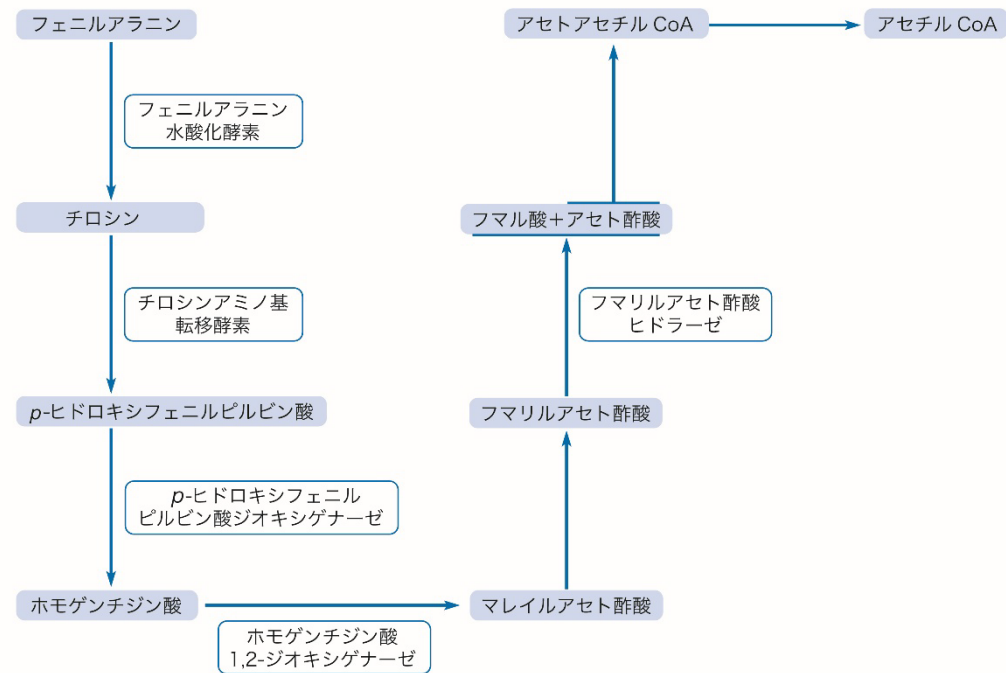
図 8-8 フェニルアラニンとチロシンの代謝系
